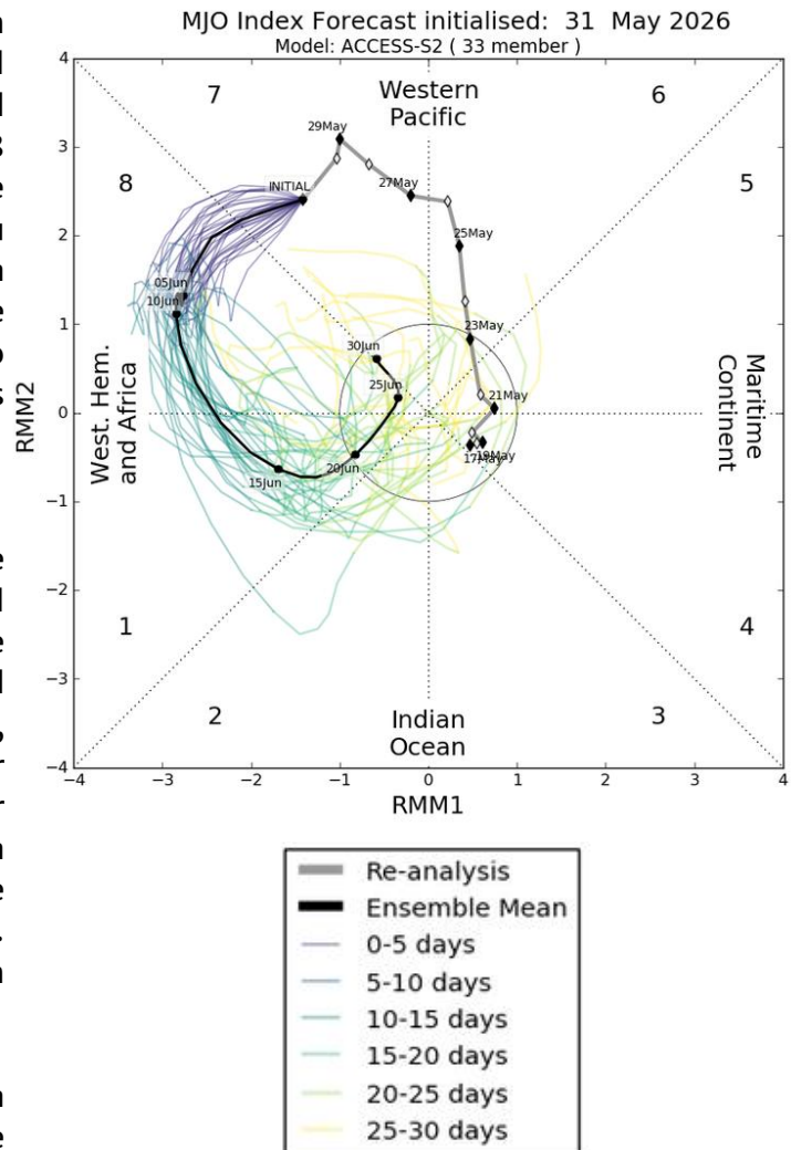
Figura 1: Pronóstico de la fase y amplitud de la Oscilación de Madden-Julian (MJO) para el mes de junio. Las proyecciones indican un tránsito por las fases 7, 8 y 1 hasta el 20 de junio. Fuente Bureau of Meteorology, Australia (BOM) consultado el 2 de junio de 2026.
