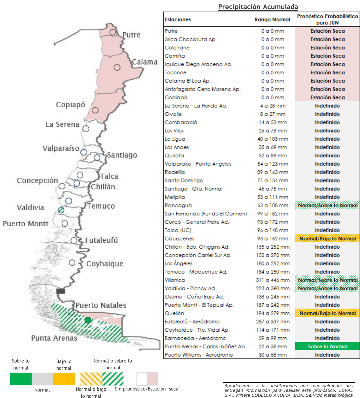
Figura 6. Pronóstico Subestacional de Precipitación acumulada para Junio 2026 , inicializado en Mayo 2026 . Se muestra el rango de precipitación más probable del mes.
